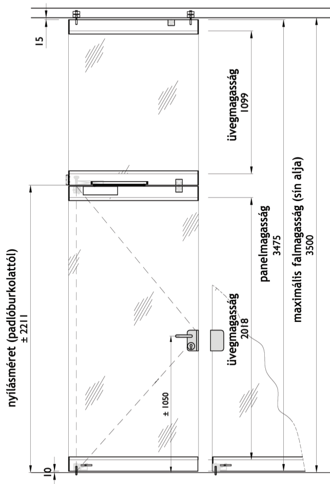
standard ajtmagasság
