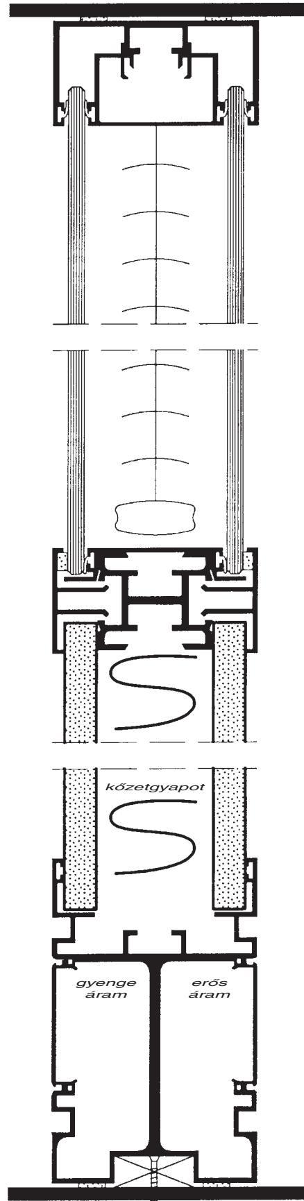
TÖMÖR PARAPETES PANEL DUPLA ÜVEGGEL, RELUXÁVAL ÉS KÁBELCSATORNÁVAL
