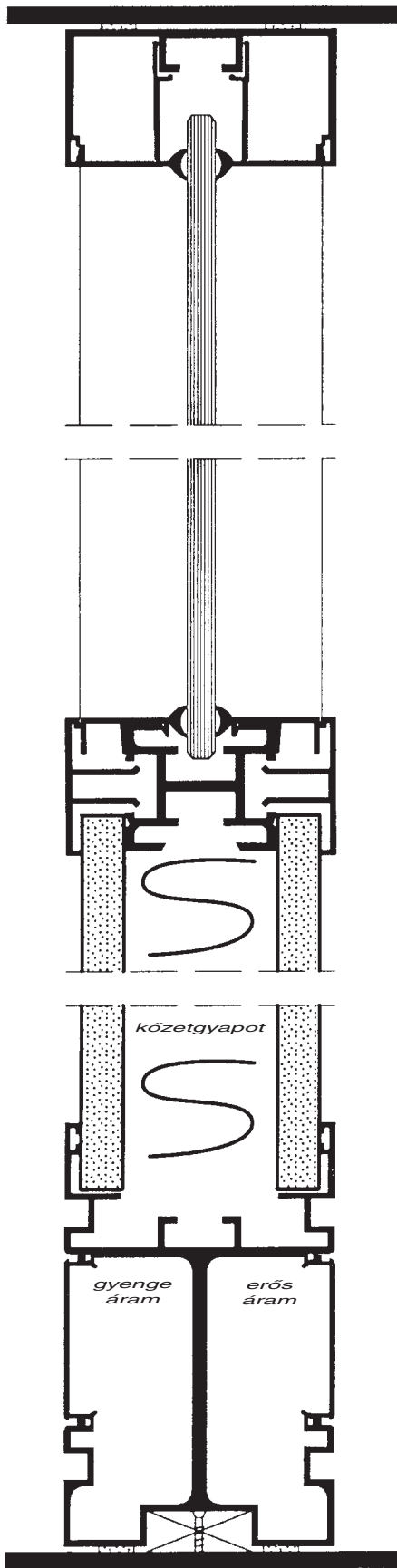
TÖMÖR PARAPETES PANEL SZIMPLA ÜVEGGEL ÉS KÁBELCSATORNÁVAL
