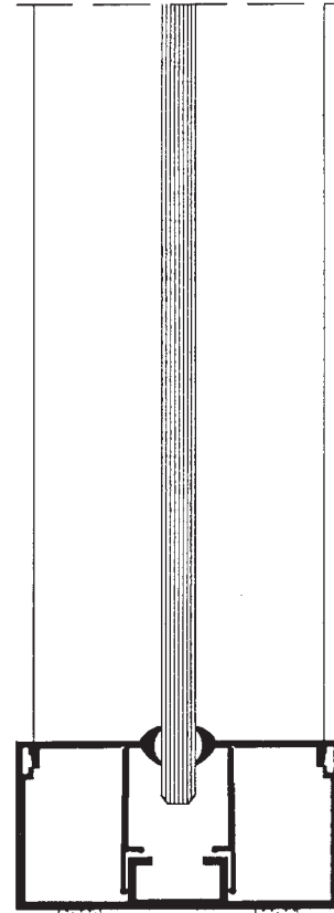
TELJES MAGASSÁGBAN SZIMPLA ÜVEGPANEL
